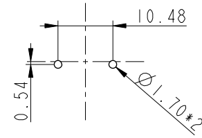
2Pin Male Connector Male Pin PCB Layout 2Pin 公接頭 PCB控孔位置尺寸圖
