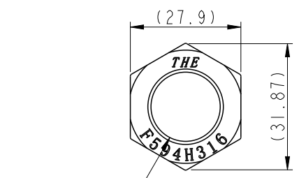
Nut
